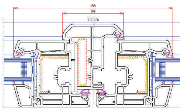
Secção Central
